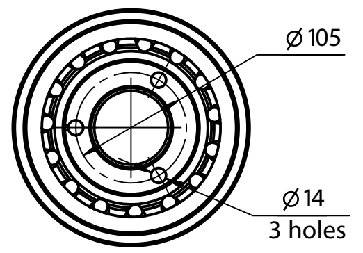
A-A (1:5)
