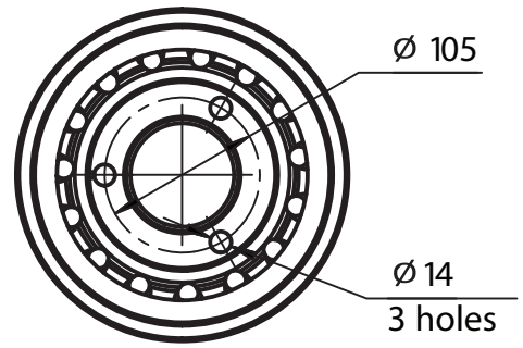
A-A (1:5)
