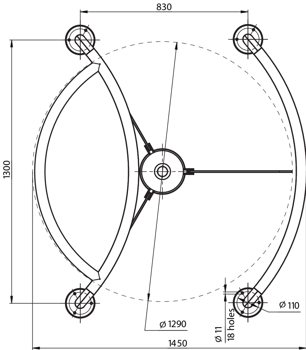
A-A (1:5)
